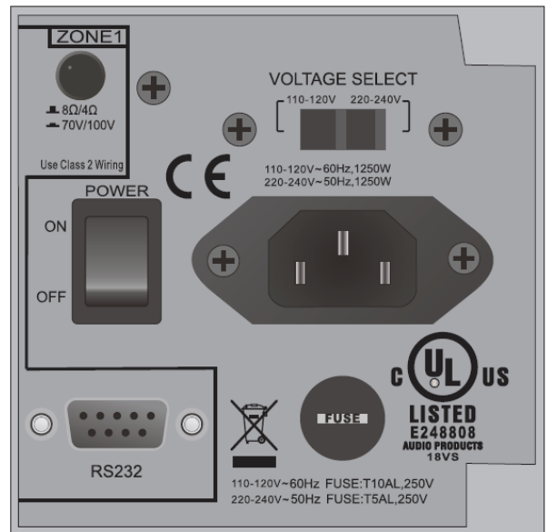
AV Voltage Select/Fuse
